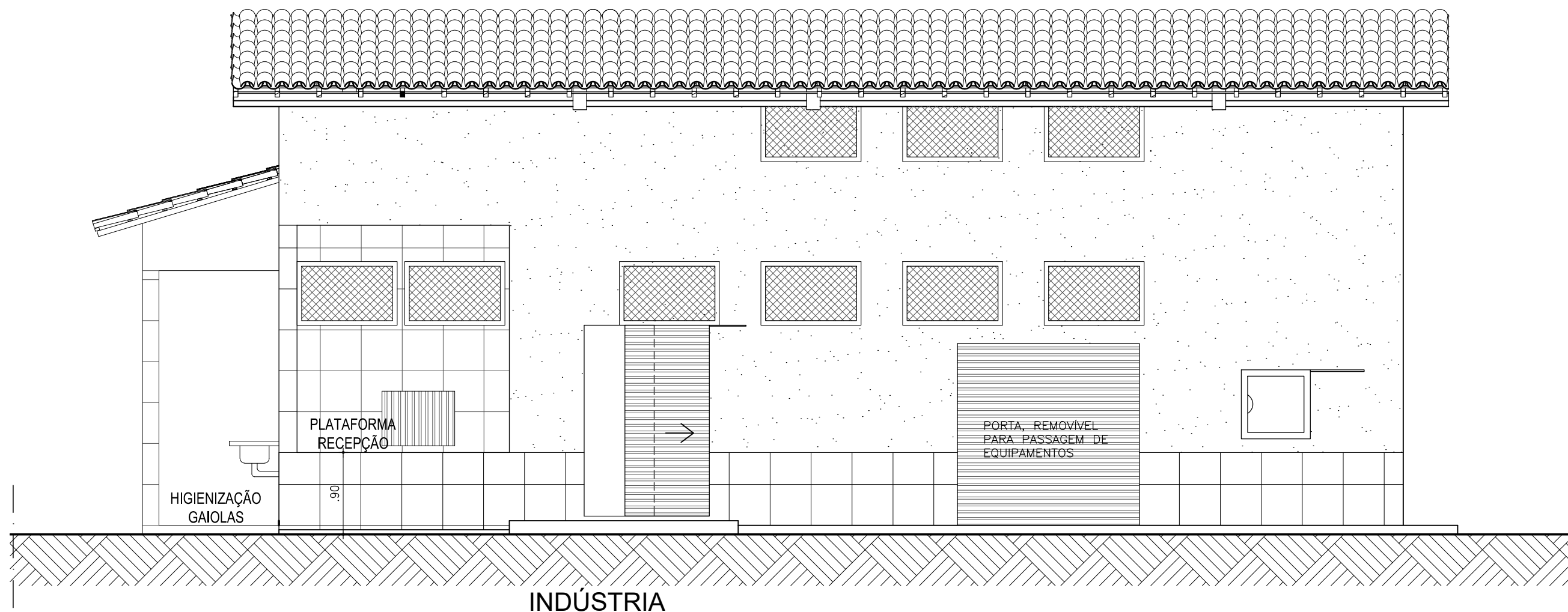
FACHADA 02 Esc. 1/50
