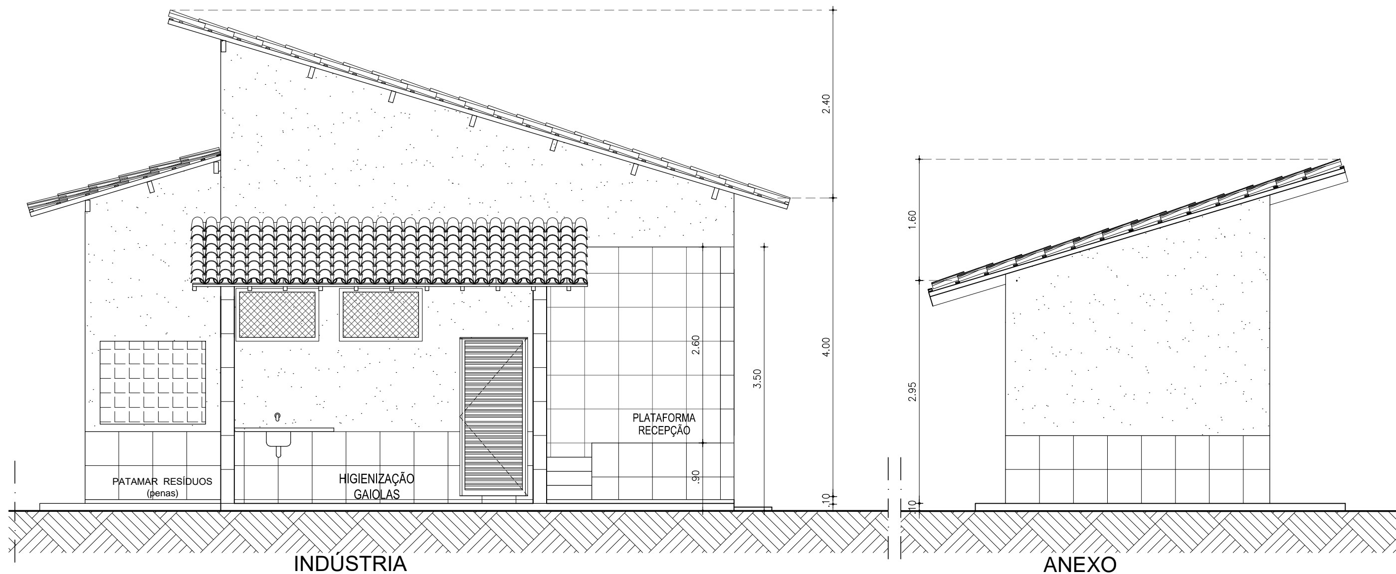
FACHADA 01 1/50
