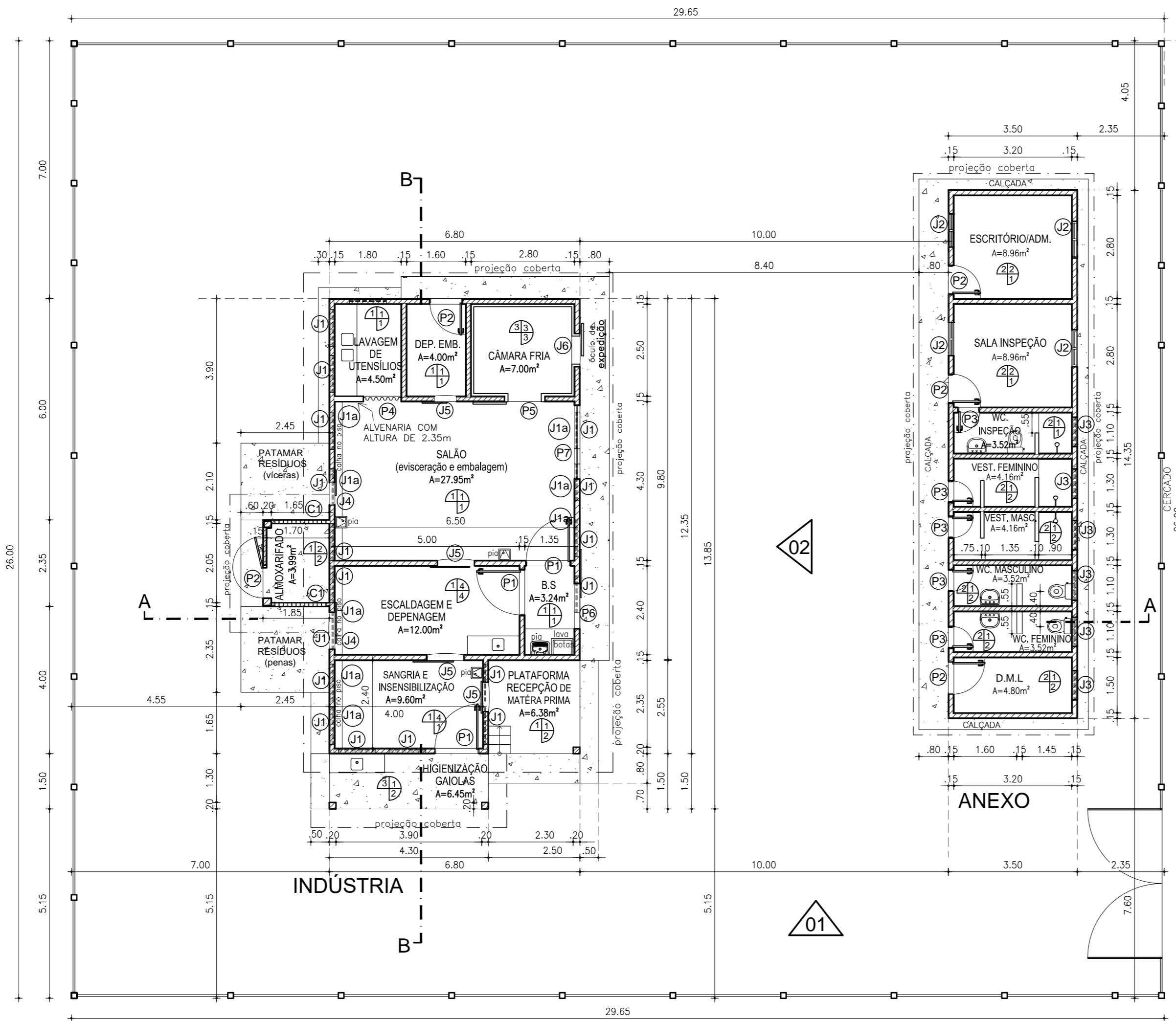
PLANTA BAIXA Esc. 1/100
